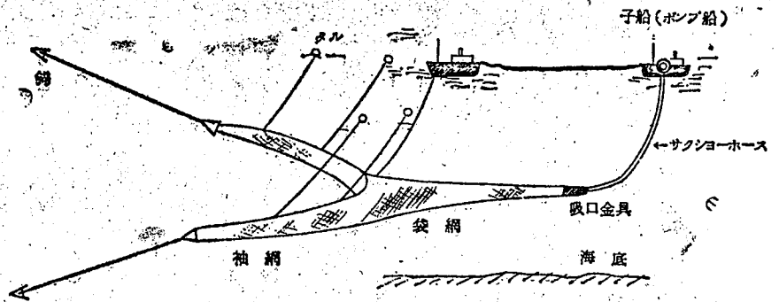
2図 Fish pump 操業見取図
