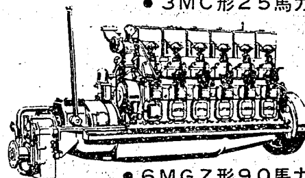
●6MGZ形90馬力
