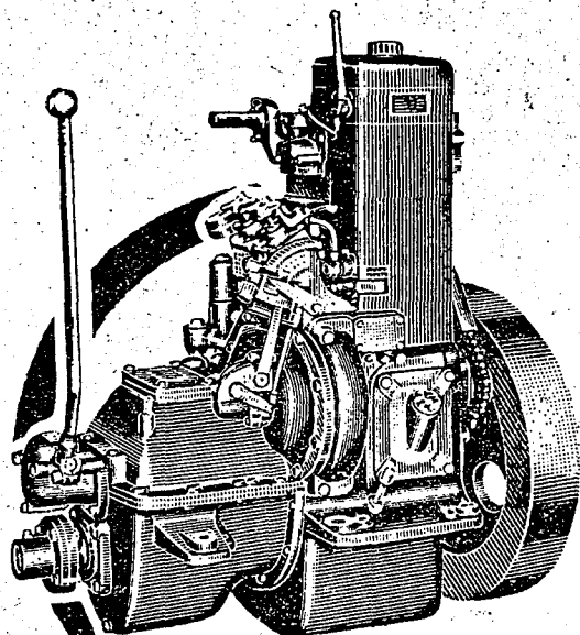
●E形(8馬力) ●EG形(10馬力)
