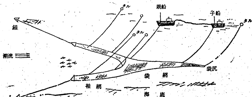
1図 袋待網操業見取図
