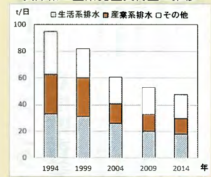
兵庫県の窒素発生負荷量の推移
